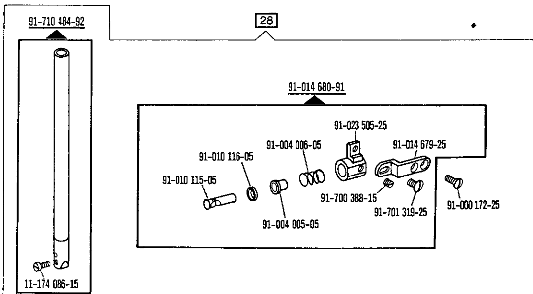
Teile zur Fadenbremse Thread retainer components Pièces du frein de fil Piezas del frenahilos
